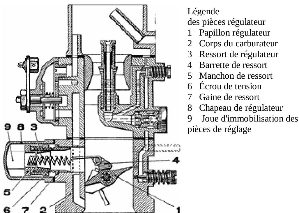
Fig. 29. - Coupe du carburateur-régulateur
