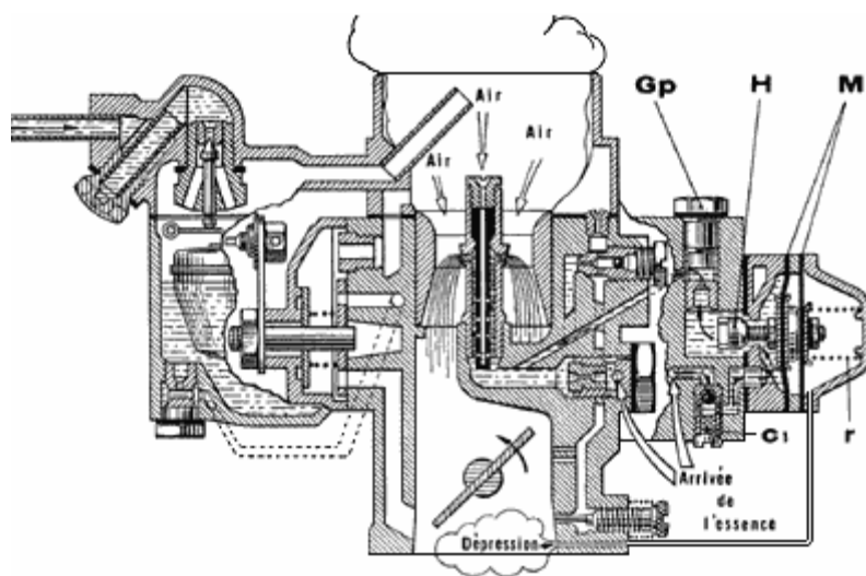
FIG. 19 : Pompe à membrane à commande pneumatique
